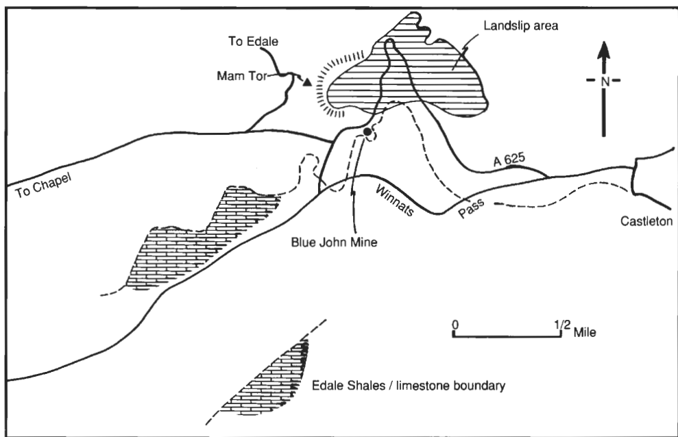
Figure 7. The Mam Tor landslide
